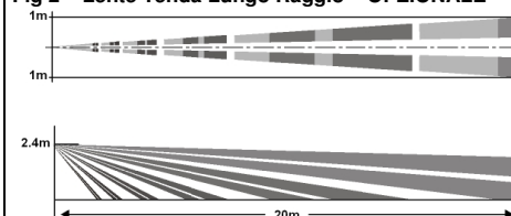
Fig. 2 – Lente Tenda Lungo Raggio – OPZIONALE
